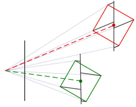
(d) para-perspective
