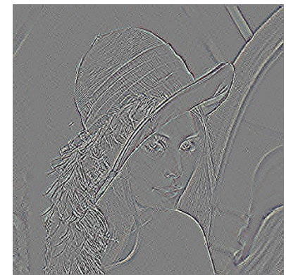
I_{yx}
